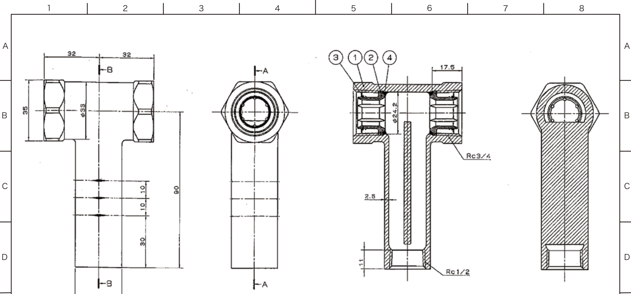
A-A断面
