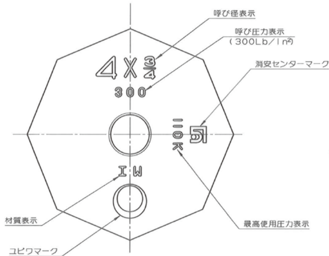
マーク配置図Bタイプ (例: 4× \frac{3}{4} )
