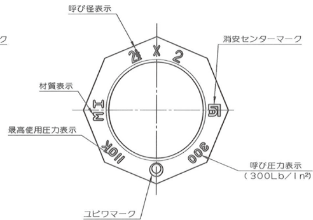
マーク配置図Aタイプ (例: 2 \frac{1}{2} ×2)
