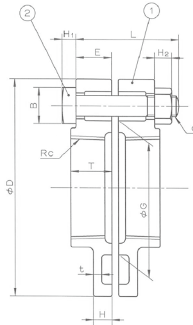
断面X-X
